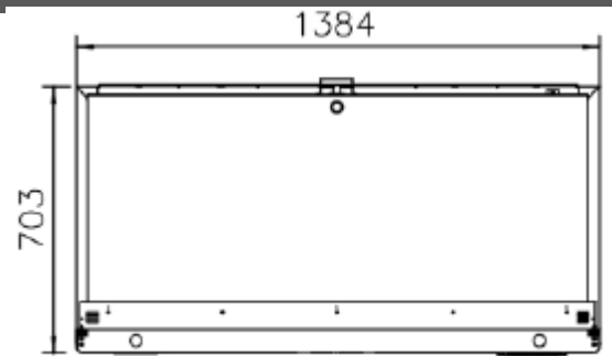
PLANTA/PLAN VIEW/DESSUS/VUE DE PROFIL
